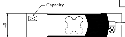
主視(Front View)
