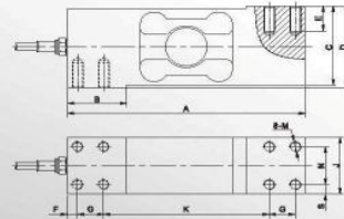
主要外形尺寸 Main Dimensions and Accessories
