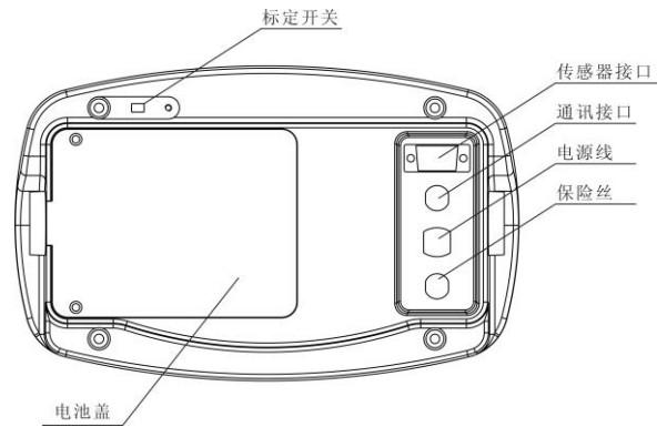
XK3118T1-F(WX) 後視圖
